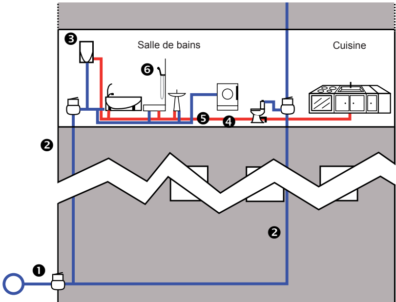
Schéma d'un réseau d'eau intérieur
